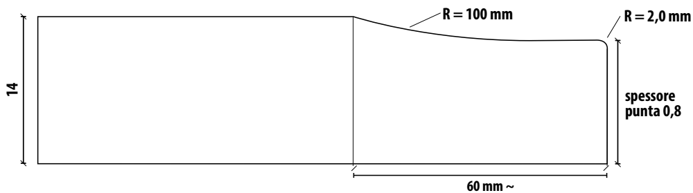
Sezione pannellatura 14 mm
