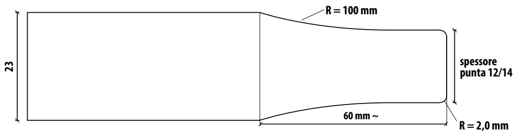
Sezione pannellatura 23 mm
