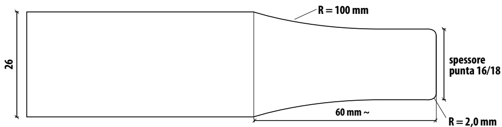
Sezione pannellatura 26 mm
