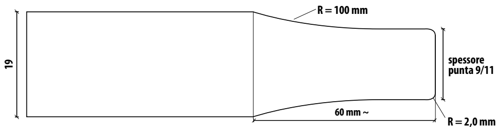
Sezione pannellatura 19 mm
