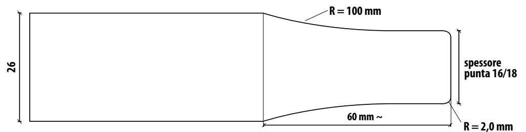
Sezione pannellatura 26 mm
