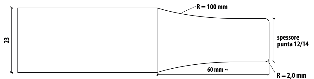
Sezione pannellatura 23 mm
